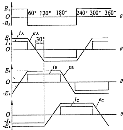
图1 电机反电势及电流波形图
